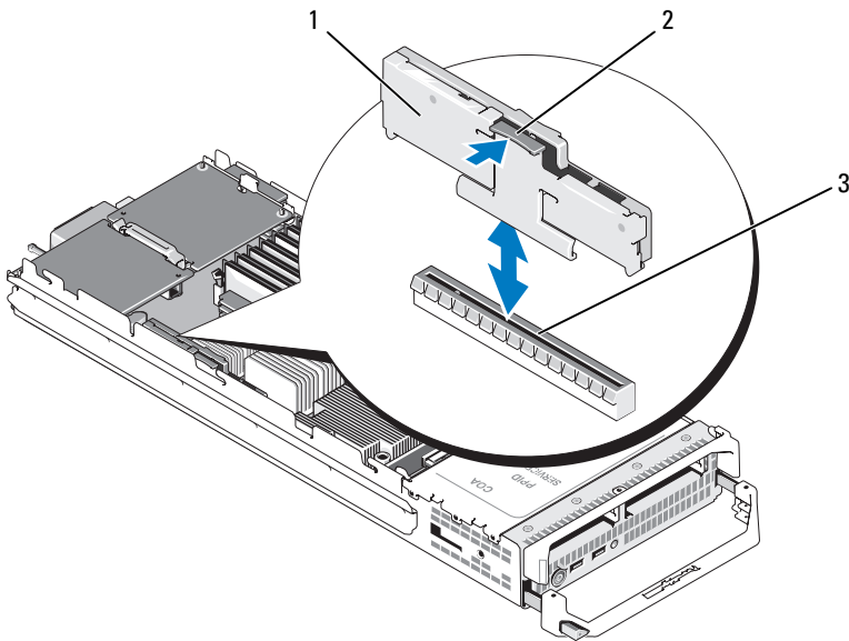
Abbildung 3-26. Grafikkarte entfernen und installieren (PowerEdge M600)
